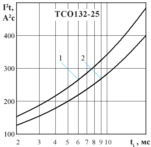
Рисунок 6 - Зависимость защитного показателя I^2t от длительности импульса тока t_1 при исходной температуре структуры T_j = 25\text{ }^\circ\text{C} (1) и максимальной температуре T_{jm} (2)
