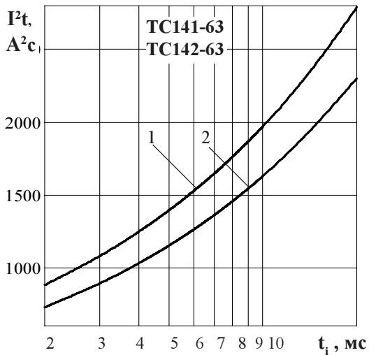
Рисунок 6 - Зависимость защитного показателя I^2t от длительности импульса тока t_1 при исходной температуре структуры T_j = 25\text{ °C} (1) и максимальной температуре T_{jm} (2)
