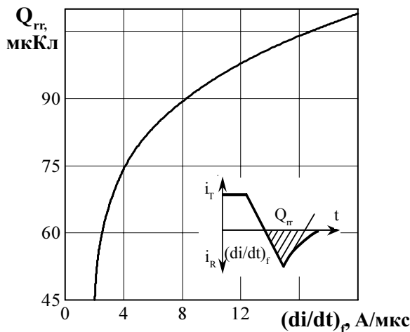
Рисунок 17 - Зависимость заряда восстановления Q_{rr} от скорости спада тока (di/dt)_r в открытом состоянии при температуре перехода T_{jm} = 125\text{ }^\circ\text{C} , U_{RM} = 100\text{ В} ; I_T = I_{T(AV)} .
