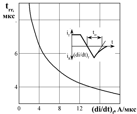
Рисунок 18 - Зависимость времени обратного восстановления t_{rr} от скорости спада тока (di/dt)_r в открытом состоянии при температуре перехода T_{jm} = 125\text{ }^\circ\text{C} , U_{RM} = 100\text{ В} ; I_T = I_{T(AV)} .
