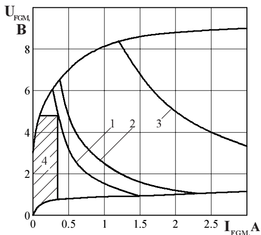
Рисунок 12 - Предельные характеристики цепи управления
