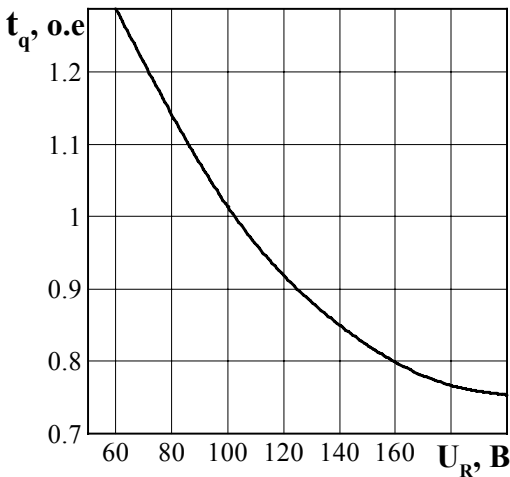
Рисунок 13 - Зависимость времени выключения t_q (о.е.) от обратного напряжения U_R при максимальной температуре перехода T_{im} = 125 \text{ }^\circ\text{C} ; I_T = I_{T(AV)} ; (di/dt)_f = 5 \text{ А/мкс} ; dU_D/dt = 50 \text{ В/мкс} ; U_D = 0,67 U_{DRM}
