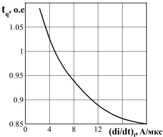
Рисунок 15 - Зависимость времени выключения t_q (о.е.) от скорости спада тока в открытом состоянии (di/dt)_f при T_{im} = 125 \text{ }^\circ\text{C} ; I_T = I_{T(AV)} ; U_R = 100 \text{ В} ; dU_D/dt = 50 \text{ В/мкс} ; U_D = 0,67 U_{DRM}
