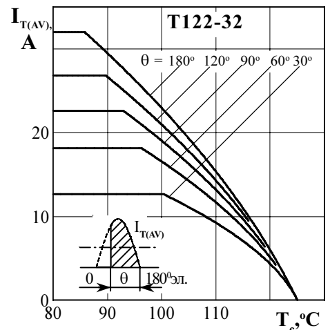
Рисунок 2 - Зависимость допустимого среднего тока в открытом состоянии I_{T(AV)} от температуры корпуса T_c для токов синусоидальной формы частоты f = 50\text{ Гц}
