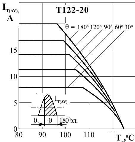
Рисунок 2 - Зависимость допустимого среднего тока в открытом состоянии I_{T(AV)} от температуры корпуса T_c для токов синусоидальной формы частоты f = 50\text{ Гц}
