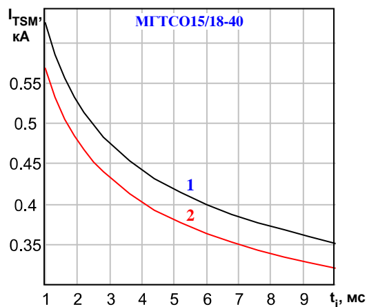
Рисунок 5: Зависимость допустимой амплитуды ударного тока в открытом состоянии I_{TSM} от длительности импульса тока t_i при исходной температуре структуры T_j = 25^\circ\text{C} (1) и максимально допустимой температуре перехода T_{jm} (2).
