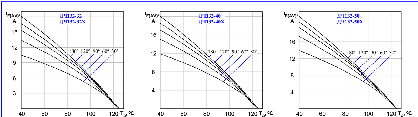
Рисунок 8: Зависимость допустимого среднего прямого тока I_{F(AV)} синусоидальной формы частотой 50 Гц при различных углах проводимости от температуры окружающей среды T_a при естественном охлаждении на ОР331-80.
