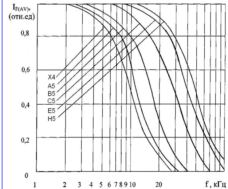
Рисунок 10: Зависимости максимально допустимого среднего прямого тока от частоты для указанных групп по времени обратного восстановления.
