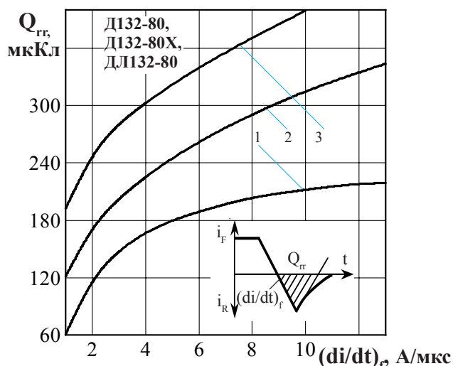
Рисунок 14 - Зависимость заряда восстановления Q_{rr} от скорости спада прямого тока (di/dt)_f при температуре перехода T_{jm} = 150\text{ }^\circ\text{C} , U_R = 100\text{ В} и при отношении амплитуды прямого тока I_F к допустимому среднему прямому току I_{F(AV)} равному: k = 0,5 (1); 1,0 (2); 1,5 (3); где k = I_F / I_{F(AV)} .
