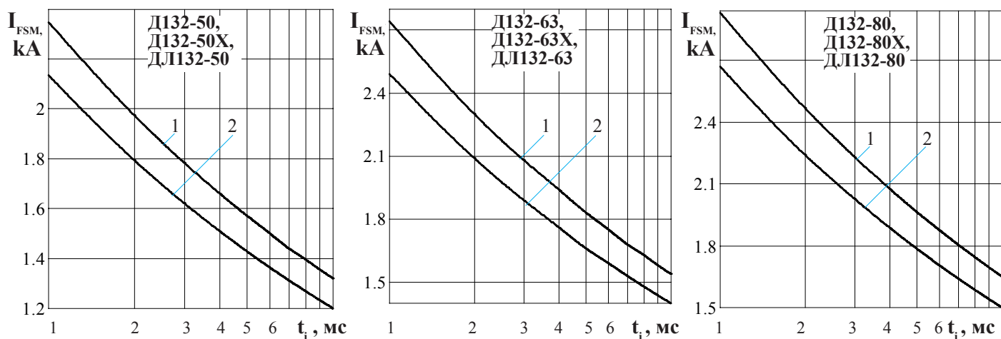
Рисунок 8 - Зависимость допустимой амплитуды ударного прямого тока I_{FSM} от длительности импульса тока t_i при исходной температуре структуры T_j = 25^\circ\text{C} (1) и максимальной температуре T_{jm} (2)
