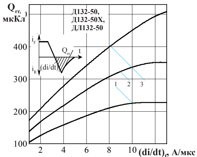
Рисунок 14 - Зависимость заряда восстановления Q_{rr} от скорости спада прямого тока (di/dt)_f при температуре перехода T_{jm} = 150\text{ }^\circ\text{C} , U_R = 100\text{ В} и при отношении амплитуды прямого тока I_F к допустимому среднему прямому току I_{F(AV)} равному: k = 0,5 (1); 1,0 (2); 1,5 (3); где k = I_F / I_{F(AV)} .
