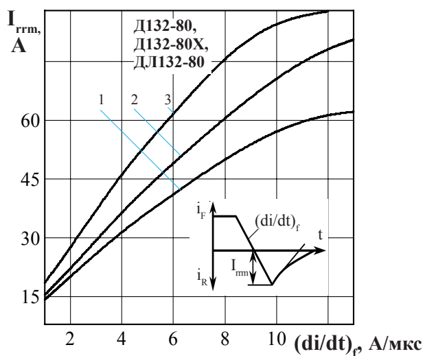
Рисунок 16 - Зависимость обратного тока восстановления I_{rrm} от скорости спада прямого тока (di/dt)_f при температуре перехода T_{jm} = 150\text{ }^\circ\text{C} , U_R = 100\text{ В} и при отношении амплитуды прямого тока I_F к допустимому среднему прямому току I_{F(AV)} равному: k = 0,5 (1); 1,0 (2); 1,5 (3); где k = I_F / I_{F(AV)} .
