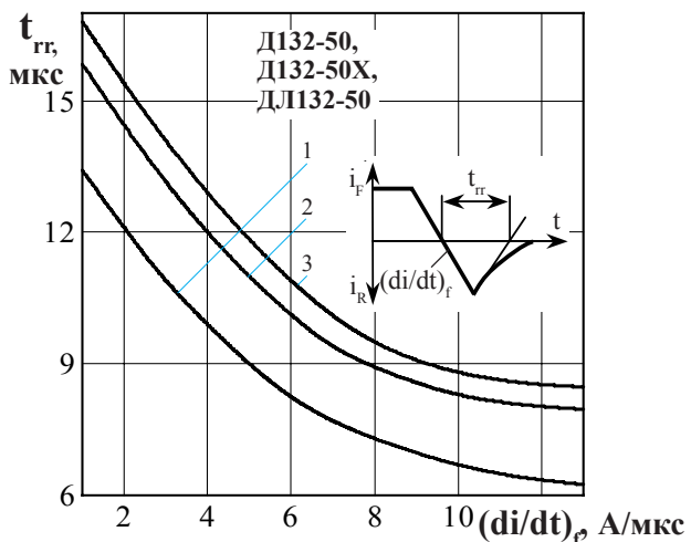
Рисунок 15 - Зависимость времени обратного восстановления t_{rr} от скорости спада прямого тока (di/dt)_f при температуре перехода T_{jm} = 150\text{ }^\circ\text{C} , U_R = 100\text{ В} и при отношении амплитуды прямого тока I_F к допустимому среднему прямому току I_{F(AV)} равному: k = 0,5 (1); 1,0 (2); 1,5 (3); где k = I_F / I_{F(AV)} .
