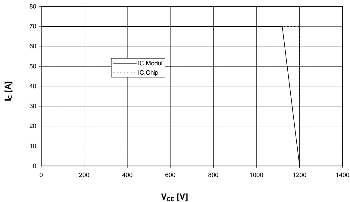
Sicherer Arbeitsbereich Wechslr. (RBSOA) I_C = f(V_{CE}) Reverse bias safe operating area Inverter (RBSOA) T_{vj} = 125^\circ\text{C}, V_{GE} = \pm 15\text{V}, R_G = 22 \text{ Ohm}
