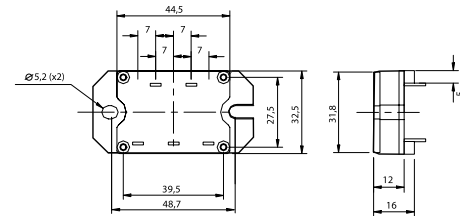
MTP-A
