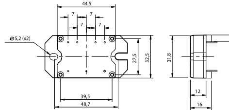
MTP-B
