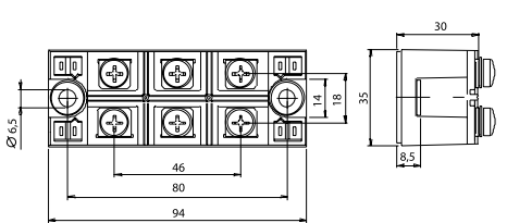
INT-A-Pak
