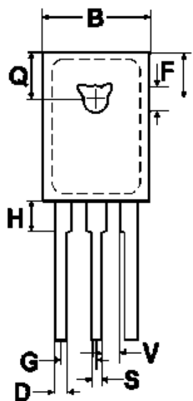
ГАБАРИТНЫЙ ЧЕРТЕЖ КОРПУСА TO-225AA (TO-126)
