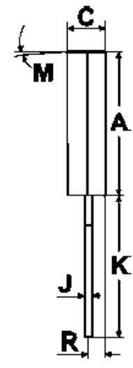
ГАБАРИТНЫЙ ЧЕРТЕЖ КОРПУСА TO-225AA (TO-126)
