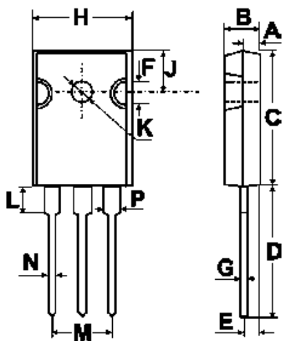
ГАБАРИТНЫЙ ЧЕРТЕЖ КОРПУСА SOT-186A
