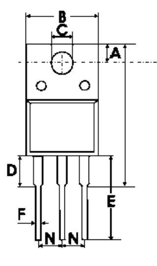
ГАБАРИТНЫЙ ЧЕРТЕЖ КОРПУСА SOT-186A
