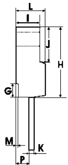
РАЗМЕРЫ КОРПУСА SOT-186A
