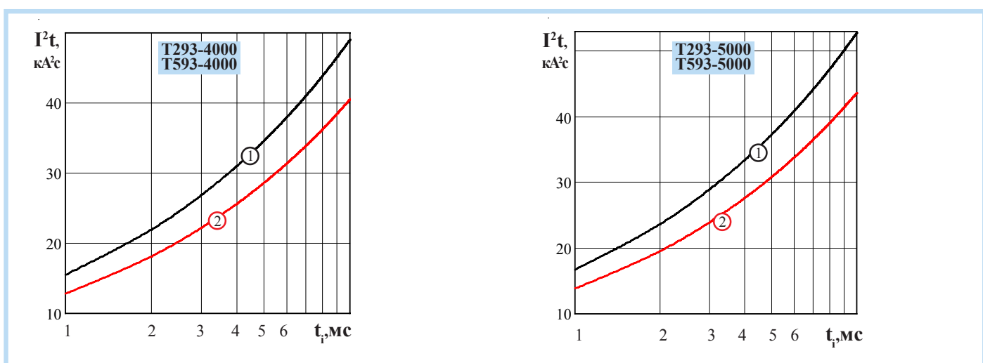
Рисунок 5 - Зависимость защитного показателя I^2t от длительности импульса тока t_p при температуре T_j = 25\text{ }^\circ\text{C} (1) и максимальной температуре перехода T_{jm} (2)
