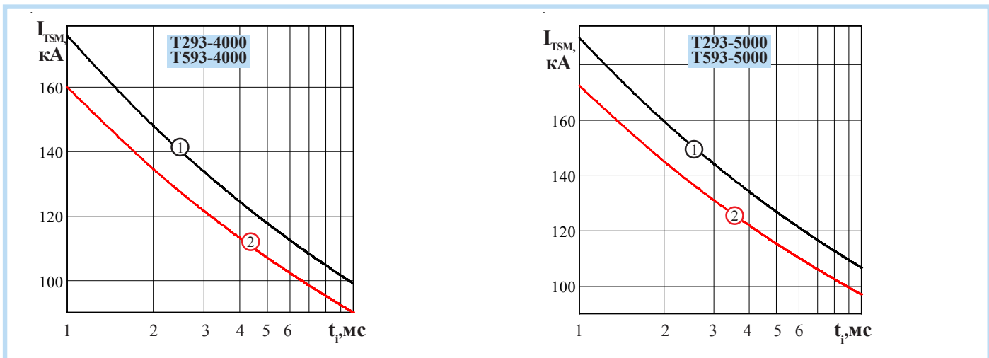
Рисунок 4 - Зависимость допустимой амплитуды ударного тока в открытом состоянии I_{TSM} от длительности импульса тока t_p при исходной температуре структуры T_j = 25\text{ }^\circ\text{C} (1) и максимальной температуре T_{jm} (2)
