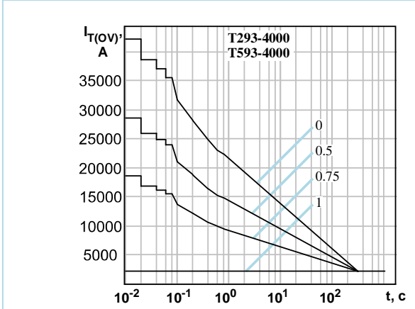
Рисунок 13: Зависимость допустимой амплитуды тока перегрузки в открытом состоянии I_{T(OV)} синусоидальной формы частотой 50 Гц от длительности перегрузки t при температуре окружающей среды 40^\circ\text{C} и при различных значениях k , равных отношению предшествующего перегрузке тока I_T к допустимому среднему току в открытом состоянии I_{T(AV)} на охладителе O193.
