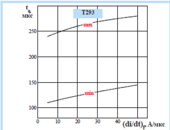
Рисунок 10 - Зависимость времени выключения t_q от скорости спада тока (di/dt)_f в открытом состоянии при T_{jm} = 125^\circ\text{C}
