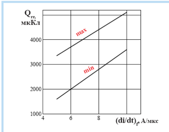
Рисунок 11 - Зависимость заряда восстановления Q_{rr} от скорости спада тока (di/dt)_f в открытом состоянии при T_{jm} = 125^\circ\text{C} ; U_R = 100\text{ В} ; I_T = I_{TAVM} .
