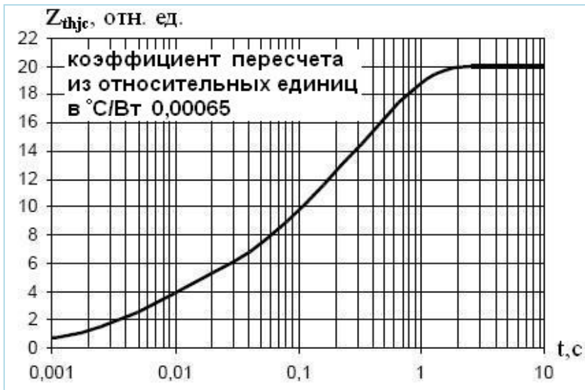
Рисунок 13: Зависимость переходного теплового сопротивления Z_{thjc} от времени t при естественном охлаждении на типовом охладителе, T_a=40^{\circ}C .
