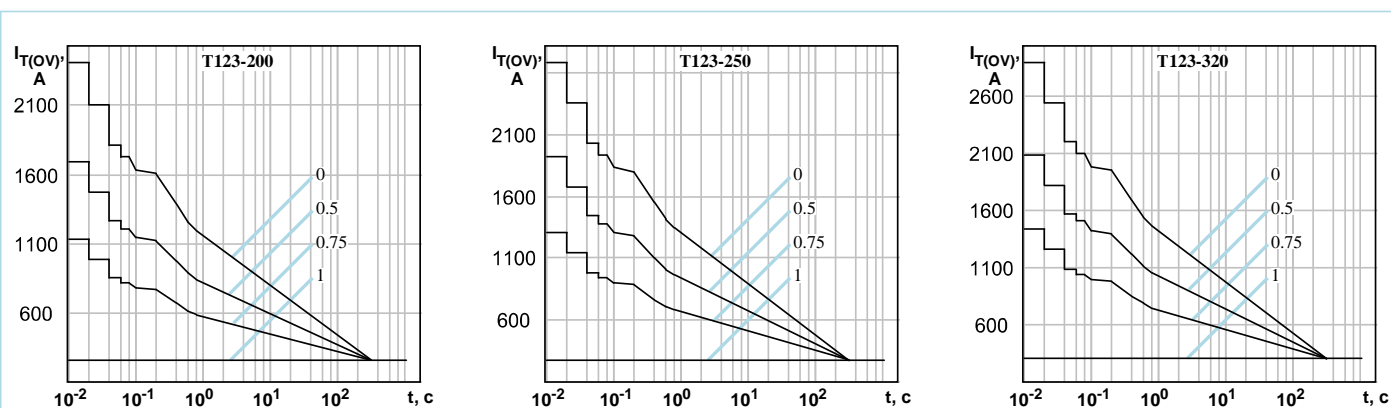
Рисунок 13: Зависимость допустимой амплитуды тока перегрузки в открытом состоянии I_{T(OV)} синусоидальной формы частотой 50 Гц от длительности перегрузки t при температуре окружающей среды 40^{\circ}\text{C} и при различных значениях k , равных отношению предшествующего перегрузке тока I_T к допустимому среднему току в открытом состоянии I_{T(AV)} на охладителе O123.
