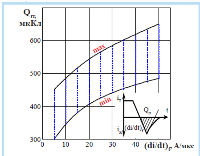
Рисунок 10 - Зависимость заряда восстановления Q_{\pi} от скорости спада тока (di/dt)_f в открытом состоянии при T_{jм} = 125^{\circ}\text{C} ; U_R = 100\text{ В} ; I_T = I_{TAVM} .
