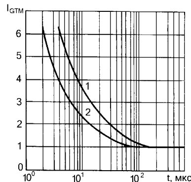
Типичные зависимости отпирющего тока управления I_{GTM} от длительности импульса управления t при температуре перехода: -60^\circ C (1), 25^\circ C (2),
