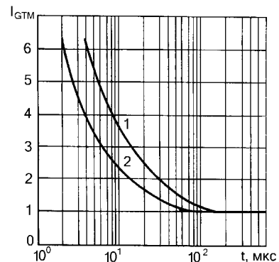
Типичные зависимости отпирающего тока управления I_{GTM} от от длительности импульса управления t при температуре перехода: -60^\circ C (1), 25^\circ C (2),
