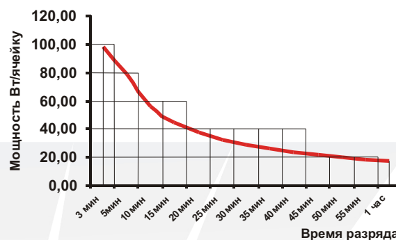
Разряд постоянной мощностью ( U_{\text{кон}}=1,7\text{ В} T=20^{\circ}\text{C} )
