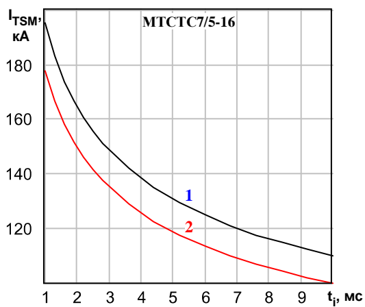
Рисунок 5: Зависимость допустимой амплитуды ударного тока в открытом состоянии I_{TSM} от длительности импульса тока t_p при исходной температуре структуры T_j = 25^\circ\text{C} (1) и максимально допустимой температуре перехода T_{jm} (2).
