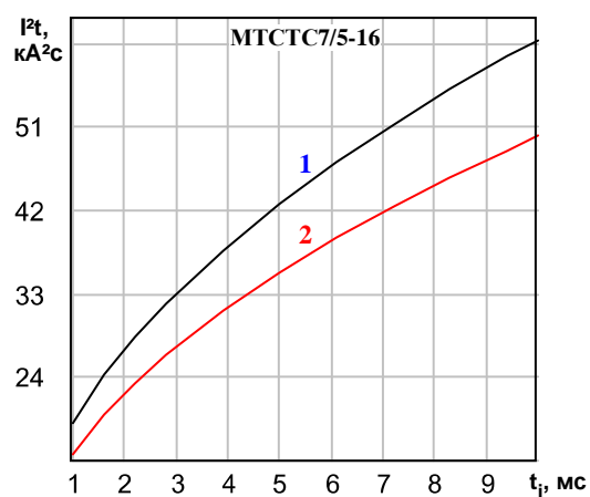
Рисунок 6: Зависимость защитного показателя I^2t от длительности импульса тока t_p при исходной температуре структуры T_j = 25^\circ\text{C} (1) и максимально допустимой температуре перехода T_{jm} (2).
