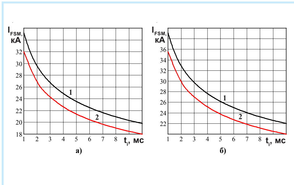
Рисунок 4 - Зависимость допустимой амплитуды ударного прямого тока I_{FSM} от длительности импульса тока t_i при исходной температуре структуры T_j = 25^\circ C (1) и максимально допустимой температуре перехода T_{jm} (2) для модулей: а) МДД14/3-500, МД16/1-500; б) МДД14/3-630, МД16/1-630.
