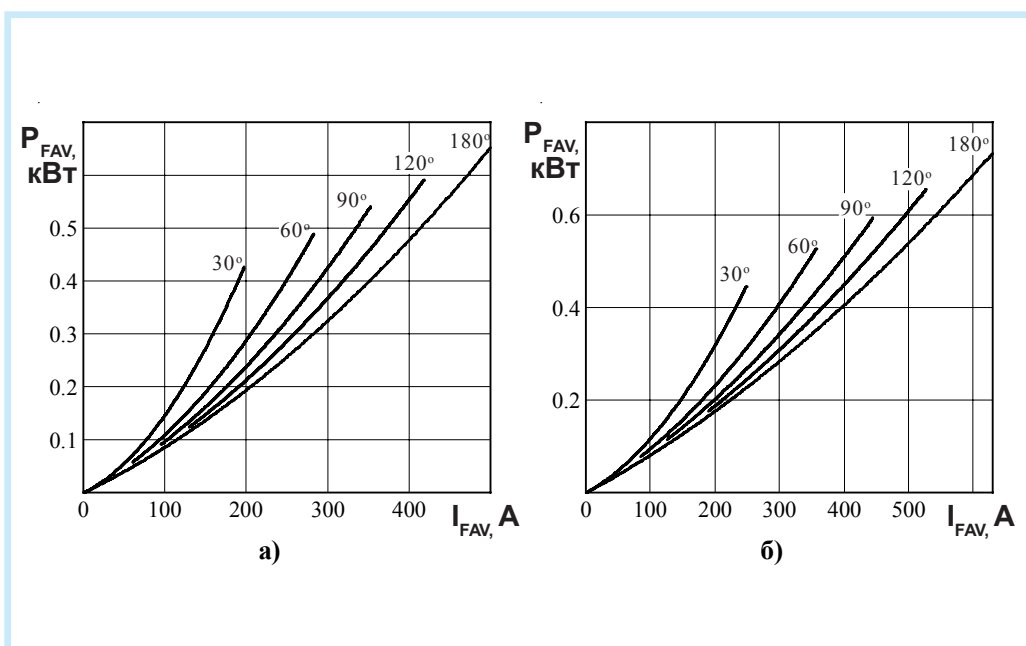
Рисунок 6 - Зависимость средней прямой рассеиваемой мощности P_{FAV} от среднего прямого тока I_{FAV} синусоидальной формы частотой 50 Гц при различных углах проводимости для модулей: а) МДД14/3-500, МД16/1-500; б) МДД14/3-630, МД16/1-630.
