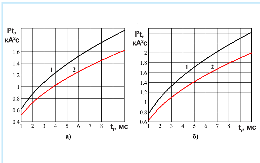
Рисунок 5 - Зависимость защитного показателя I^2t от длительности импульса тока t_i при температуре T_j = 25^\circ C (1) и максимально допустимой температуре перехода T_{jm} (2) для модулей: а) МДД14/3-500, МД16/1-500; б) МДД14/3-630, МД16/1-630.
