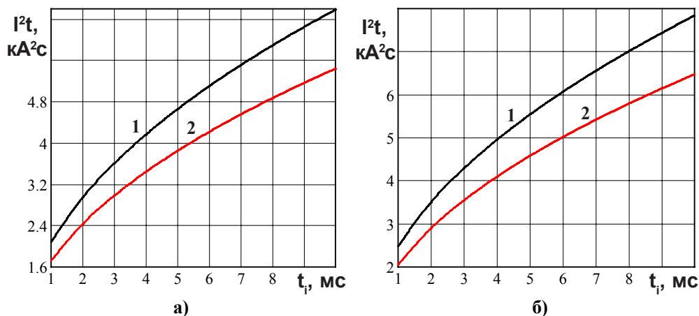
Рисунок 5 - Зависимость защитного показателя I^2t от длительности импульса тока t_i при температуре T_j = 25^\circ C (1) и максимально допустимой температуре перехода T_{jm} (2) для модулей: а) МДД13/3-1000, МДД13/4-1000, МДД13/5-1000, МД17/1-1000; б) МДД13/3-1250, МДД13/4-1250, МДД13/5-1250, МД17/1-1250.
