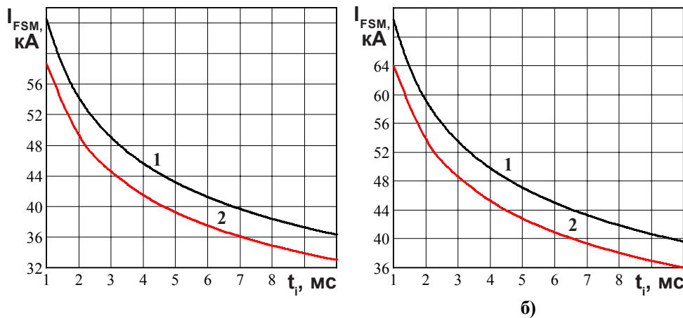
Рисунок 4 - Зависимость допустимой амплитуды ударного прямого тока I_{FSM} от длительности импульса тока t_i при исходной температуре структуры T_j = 25^\circ C (1) и максимально допустимой температуре перехода T_{jm} (2) для модулей: а) МДД13/3-1000, МДД13/4-1000, МДД13/5-1000, МД17/1-1000; б) МДД13/3-1250, МДД13/4-1250, МДД13/5-1250, МД17/1-1250.
