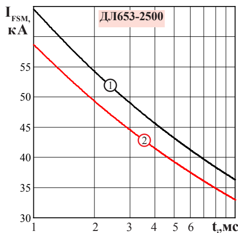
Рисунок 4 - Зависимость допустимой амплитуды ударного прямого тока I_{FSM} от длительности импульса тока t_i при температуре T_j = 25^\circ\text{C} (1) и максимальной температуре перехода T_{jm} (2)
