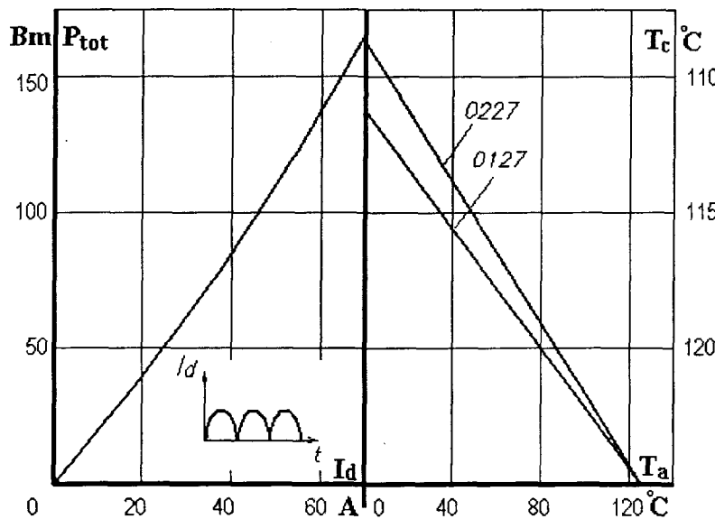
Рис. 2. 31.* Зависимость допустимой суммарной рассеиваемой мощности и допустимого выпрямленного тока двух модулей МТТ4/3 - 100 на охладителях О127 и О227 от температуры окружающей среды и температуры корпуса при естественном охлаждении
