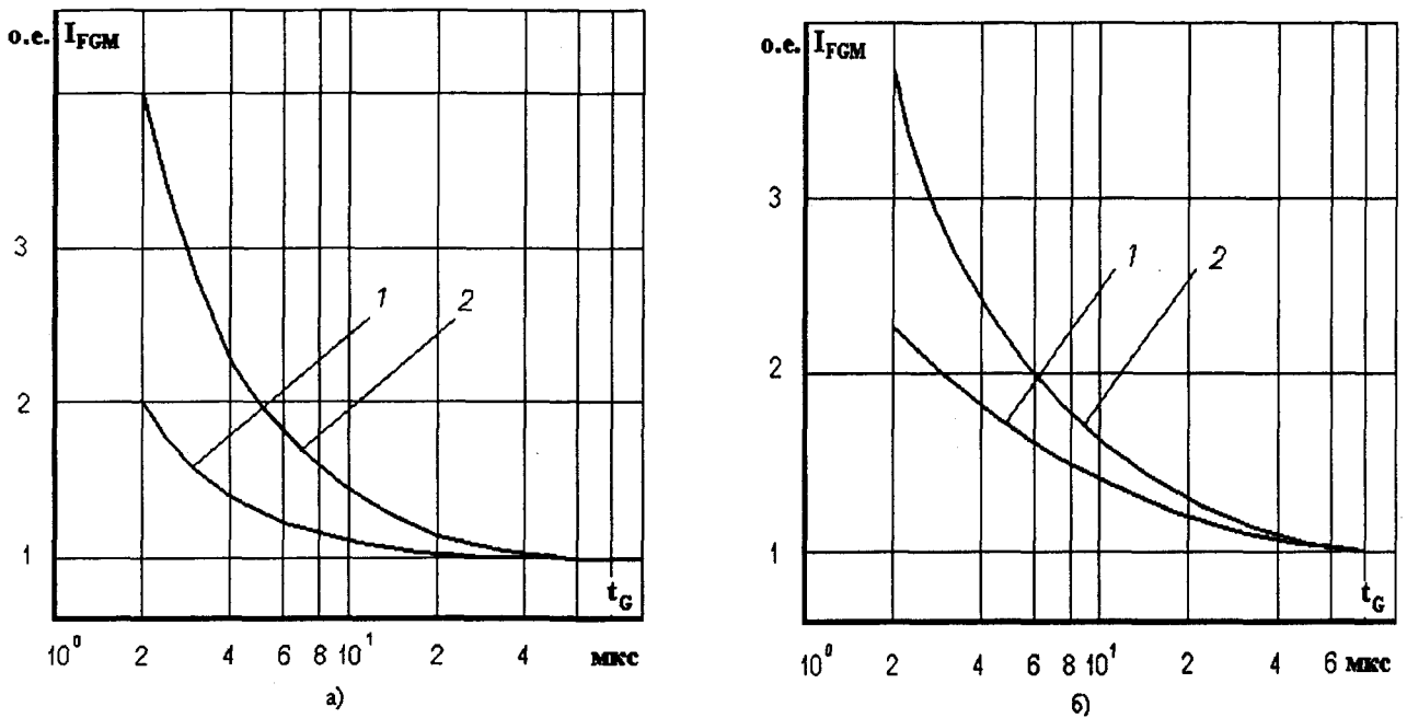
Рис. 2. 14. Зависимость отпирющего импульсного тока управления I_{GGM} от длительности управляющего импульса t_G при температуре перехода T_j = 25 °С (1) и минимально допустимой температуре T_{jmin} (2), U_D = 12 В
