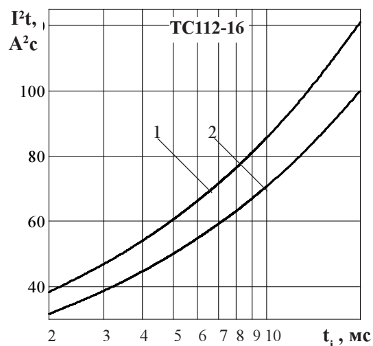
Рисунок 6 - Зависимость защитного показателя I^2t от длительности импульса тока t_i при исходной температуре структуры T_j = 25\text{ }^\circ\text{C} (1) и максимальной температуре T_{jm} (2)
