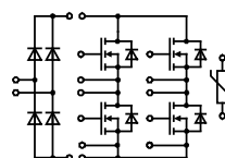
X104 V2-Pack
