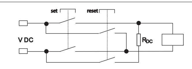
Работа при DC
