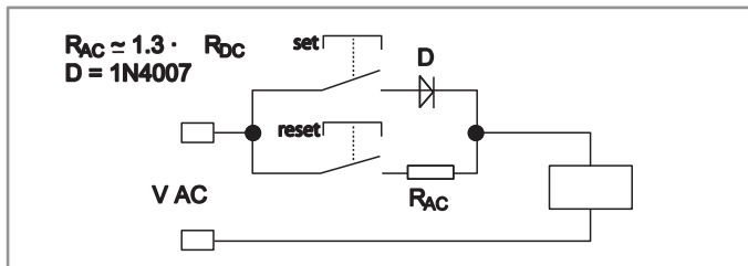
Работа при AC
