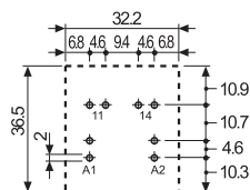
Вид сбоку
