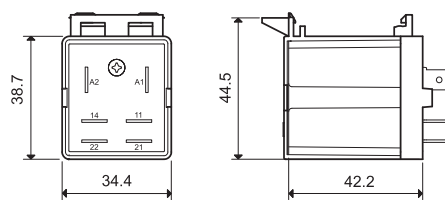
065.08 с реле
