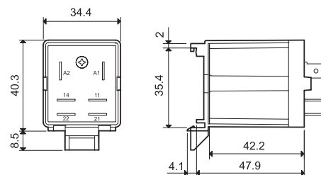
065.07 с реле
