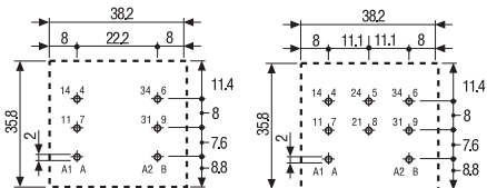
62.22 - 0300 Вид сбоку
