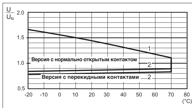
R 56 - Отношение рабочего диапазона для AC к температуре окр. среды - Реле с 4 перекидными или 4 НО контактами
