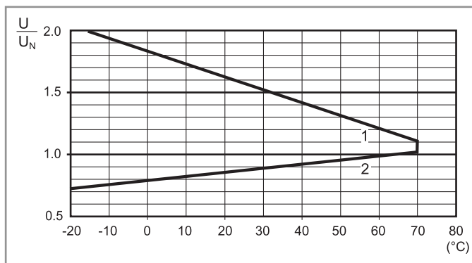
R 56 - Отношение рабочего диапазона для DC к температуре окр. среды - Реле с 4 перекидными контактами
