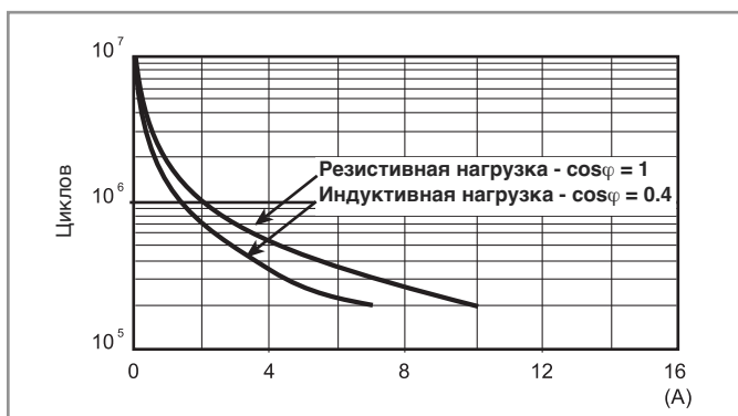
F 55 - Электрическая долговечность (AC) при ном. нагрузке Реле с 2 и 3 перекидными контактами
