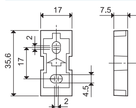
Блок маркировок для типа 15.81, пластик, 72 знаков, 6x12 мм
