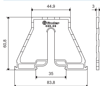
Разделитель для щитового монтажа для типа 15.81
